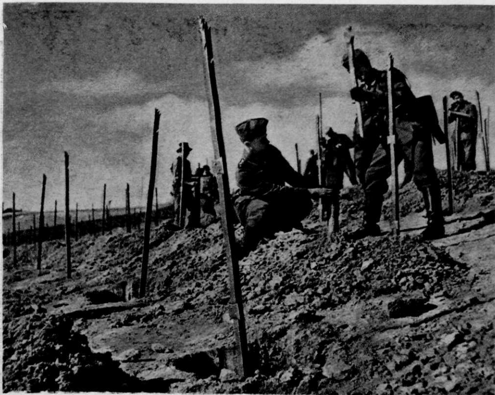
Afb. 8. Palen voor draadversperringen worden in den rotsgrond verankerd.
