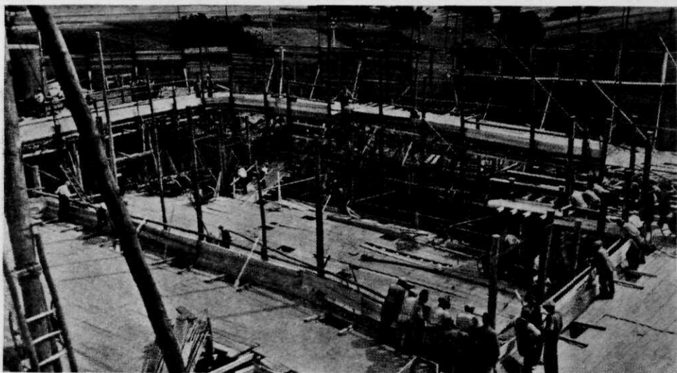
Afb. 2. Bouw van een pantserwerk in de Siegfriedlinie.
