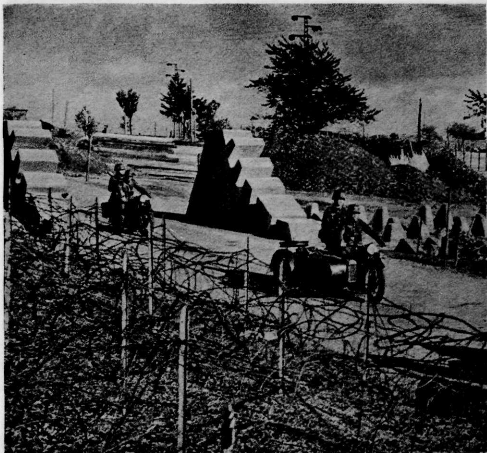
Afb. 6. Waar de linie van betonnen hindernissen tegen pantserwagens een weg snijdt, vormen boogvormige betonnen bouwwerken, waarin spoorstaven gelegd worden, een afsluiting van den weg.
