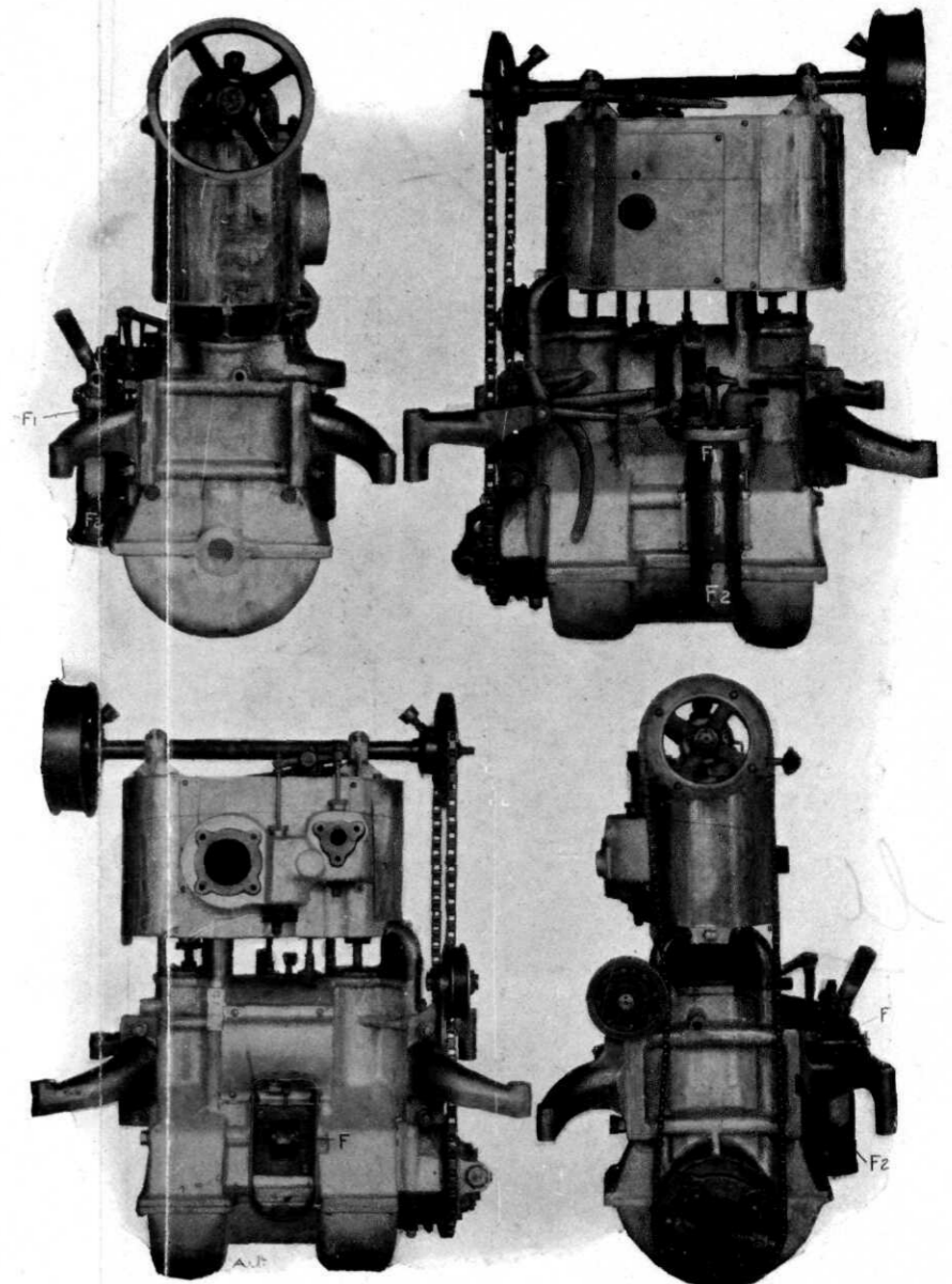
FIG. V, VI, VII, VIII. Afbeeldingen van de 30 H.P. White machine van elke zijde afzonderlijk gezien.
