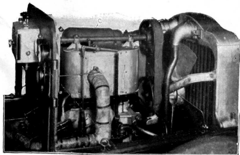
FIGUUR III. Afbeelding van den zijkant der 30 H.P. White machine in de chassis opgesteld.
