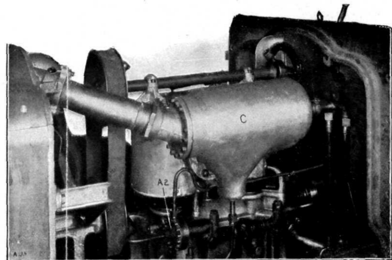
FIGUUR IV. Afbeelding van den binnenkant der 30 H.P. White machine in de chassis opgesteld.
