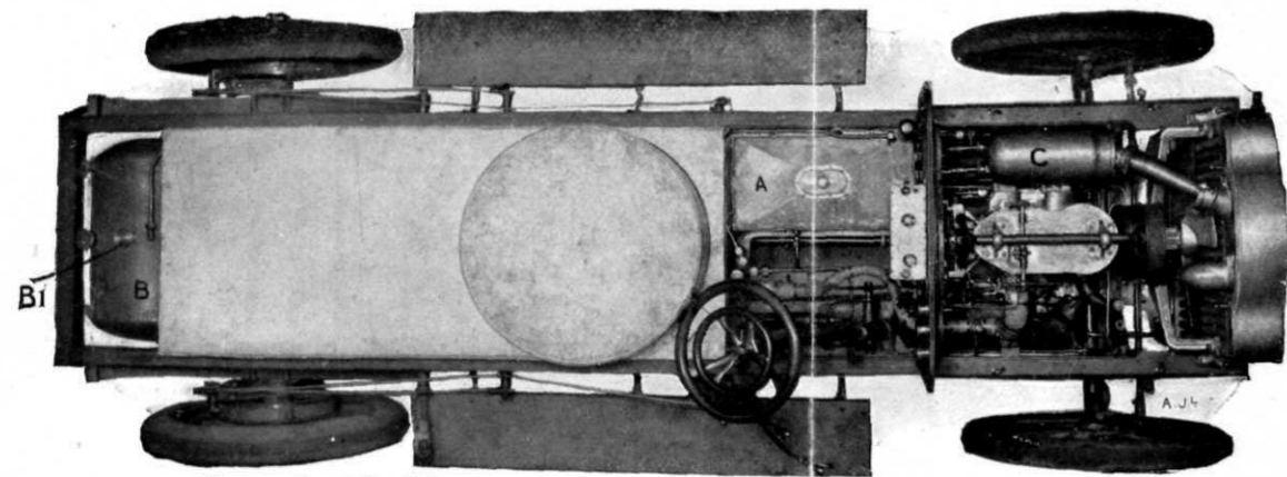
FIGUUR I. Afbeelding van de 30 H.P. White chassis van den bovenkant.
