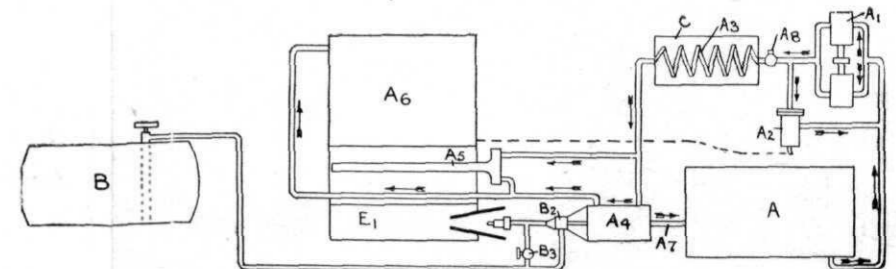
FIGUUR IX. Doorsnede van het verbeterde White Steam-stelsel tot regeling van watertoevoer met de gewijzigde thermostaat-controle.
