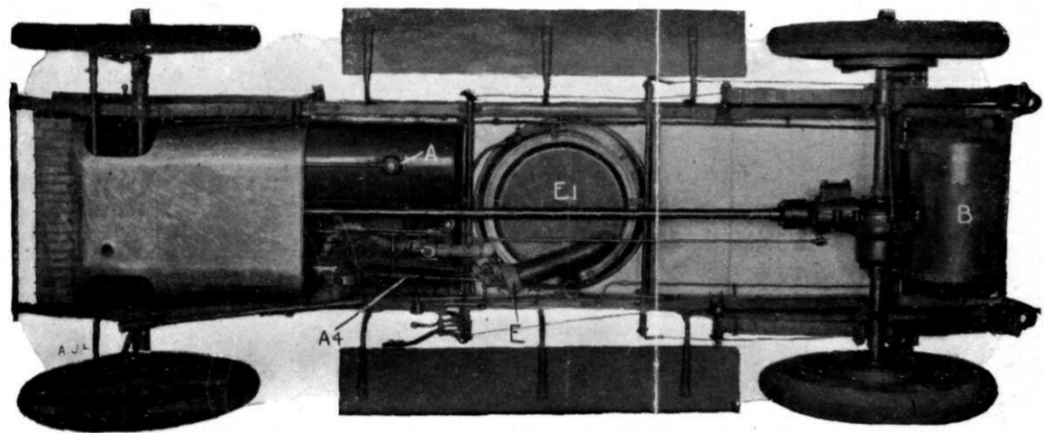
FIGUUR II. Afbeelding van de 30 H.P. White chassis van den onderkant.
