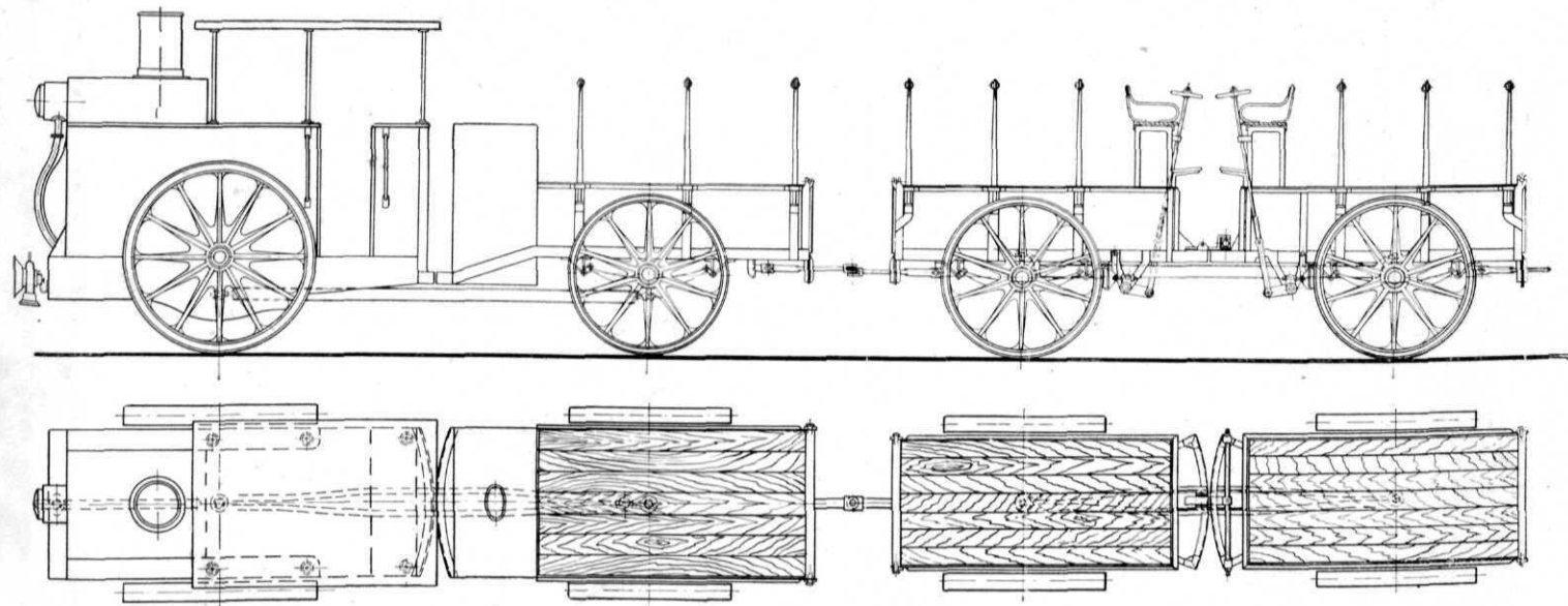
FIGUUR 2. Algemeene inrichting van den Freibahntrein.
