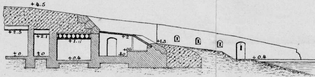
Fig: 4 Doorsnede volgens E.F. (1:200)
