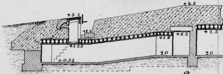
Fig: 4 Doorsnede volgens E.F. (1:200)
