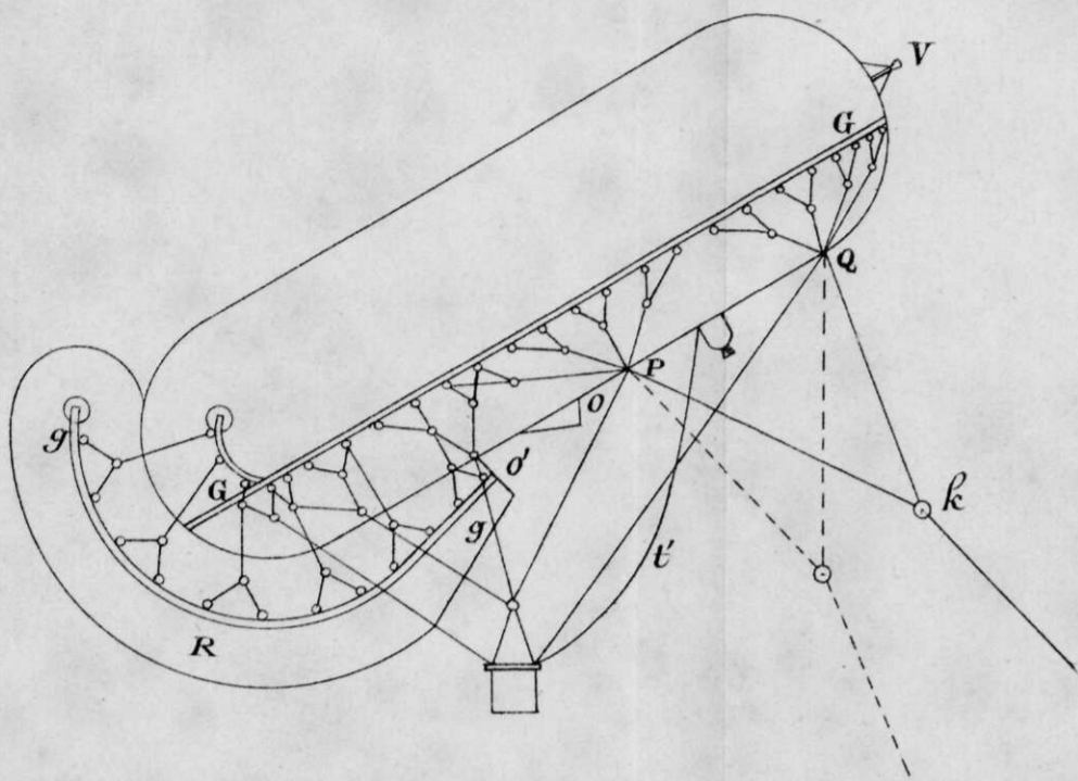
Fig. 3. Gierbeweging
