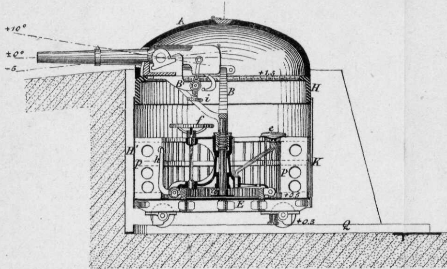
Fig. 2. (1:30)
