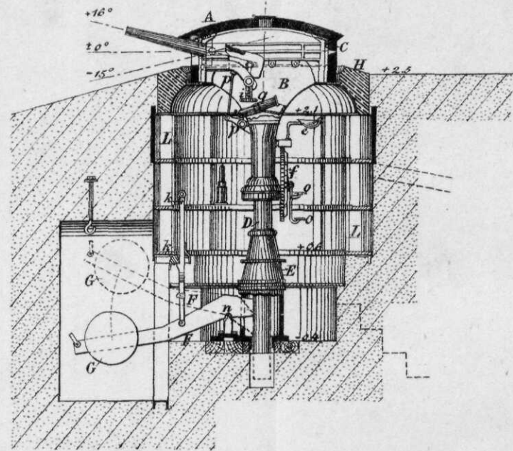
Fig. 4. (1:60)
