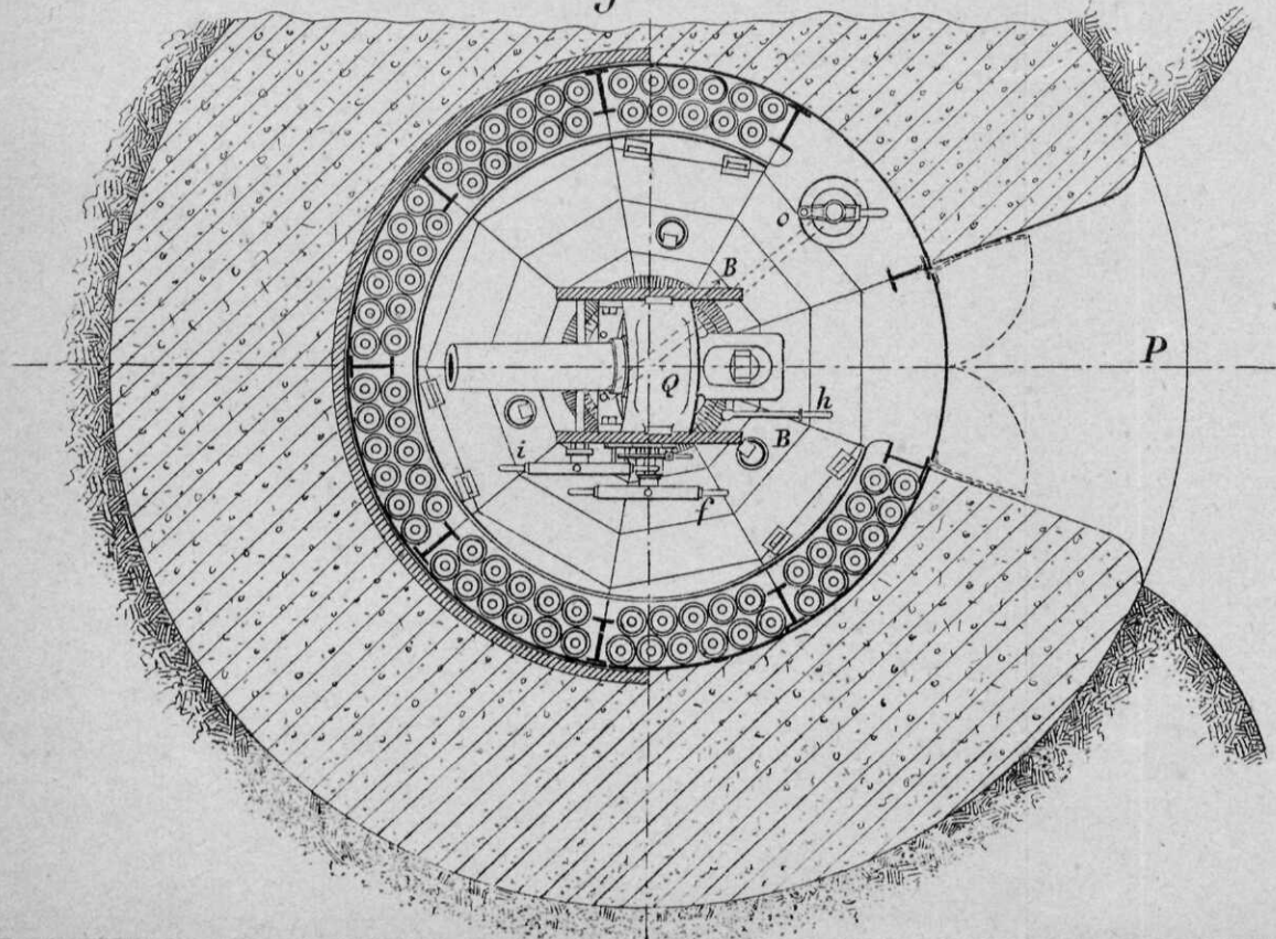
Fig. 2. (1/2).
