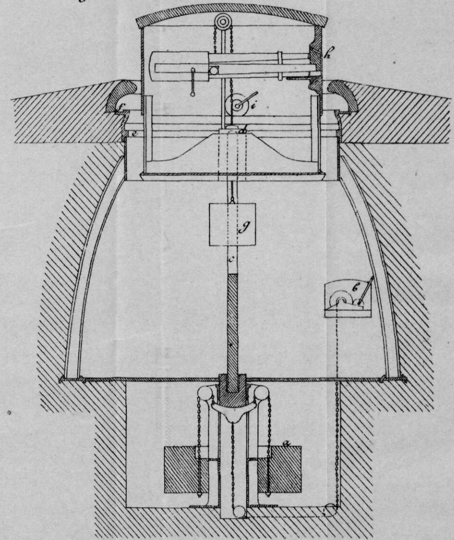
Fig. 3. Pantsering voor revolverkanonnen van 53 m M.
