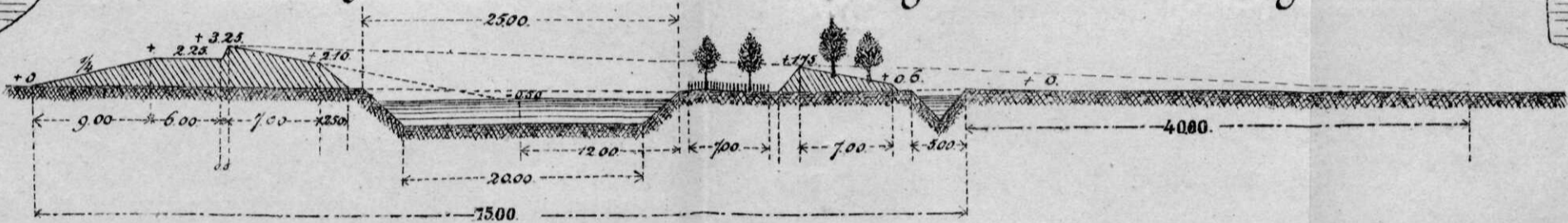
Fig. 3. (1/500) Profiel over een bestaanden boogen fortwal met glacis.
