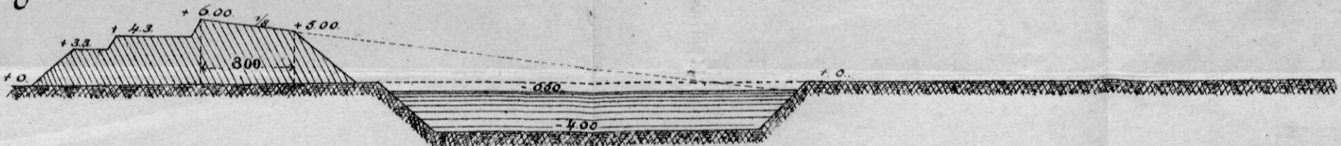
Fig. 6. (1/500) Gewijzigd profiel Fig. 5.
