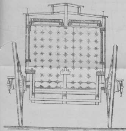
FIG.3.STANDGEZICHT VAN ACHTEREN. (1:25).
