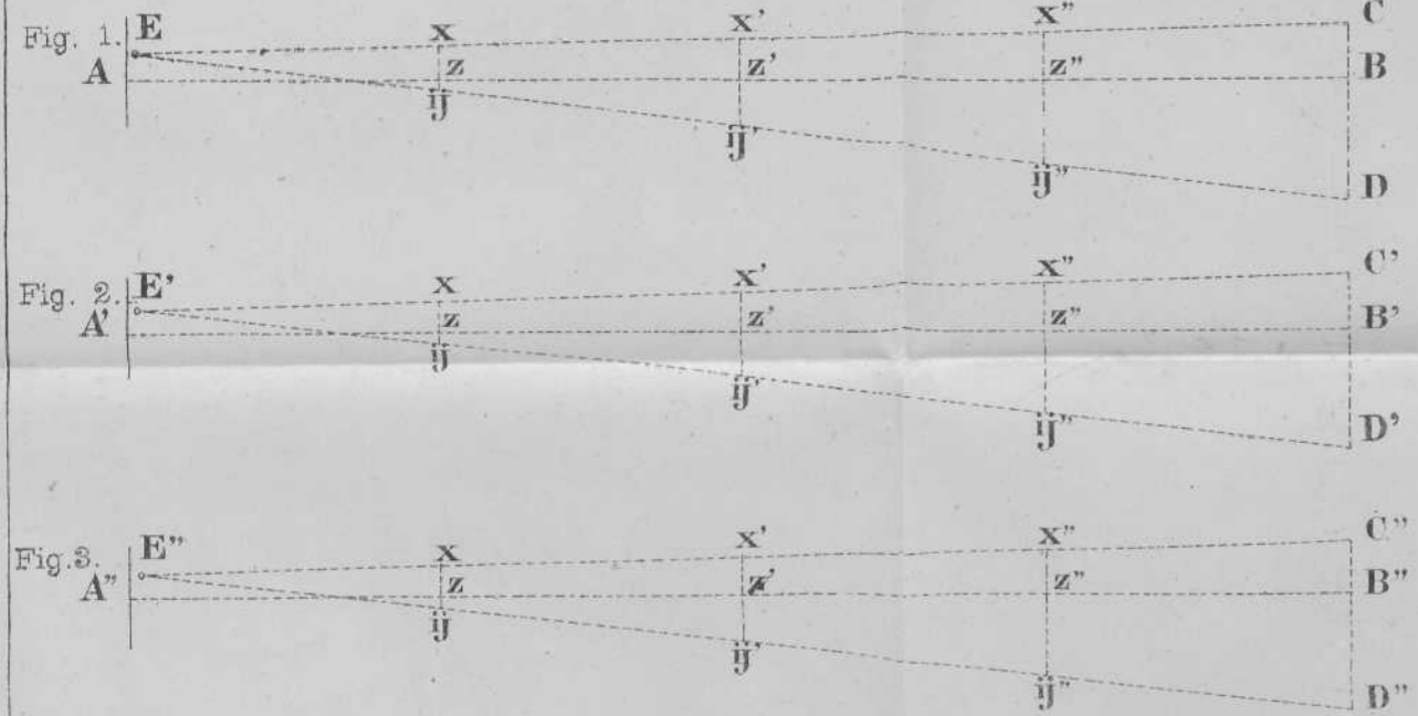
Graphische schetsen van het waarnemingsveld der spinnen E, E' en E'' van de evenwijdige open schietbanen AB, A'B' en A''B'.
