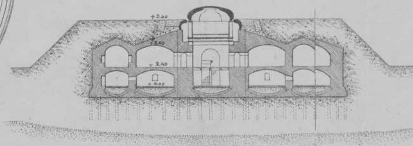
FIG. 4. DOORSNEDE AB. 1:500.
