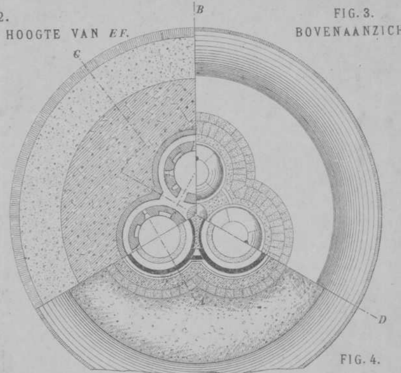
FIG. 4. DOORSNEDE OP DE HOOGTE VAN GH.
