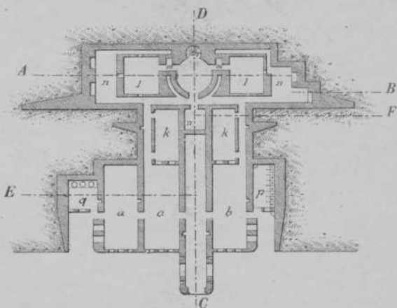
FIG. 3. BOVENVERDIEPING. 1:750.
