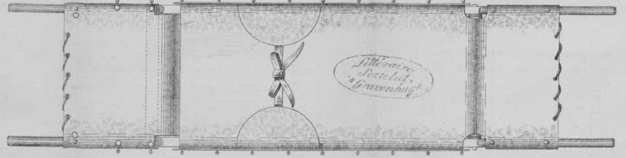
FIG.10.DE BRANCARD VAN TER ZIJDE. (1:10). (Een der draaizarmen in- en een uitgeschoven).
