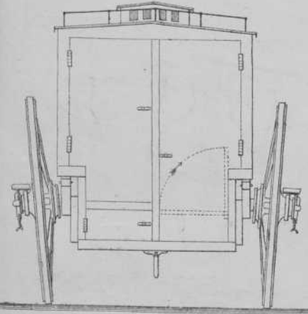
FIG.3.STANDGEZICHT VAN ACHTEREN. (1:25).
