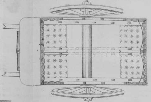
FIG.5.PLATTE GROND DER KAR VOOR 4 ZITZENDE LIJDERS INGERICHT. (1:25).
