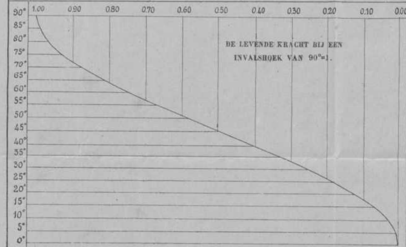
GRAPHISCHE VOORSTELLING DER LEVENDE KRACHT VAN PROJECTIELEN BIJ VERSCHILLENDE INVALSHOEKEN.
