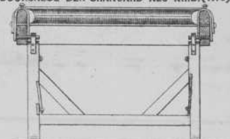
FIG.12.DE BRANCARD ALS KRIB VAN VOREN GEZIEN. (1:10).
