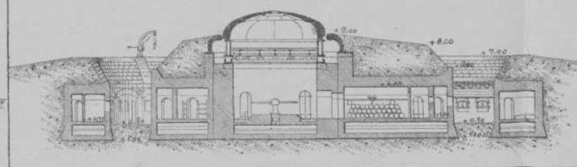
FIG. 8. DOORSNEDE GH. 1:500.
