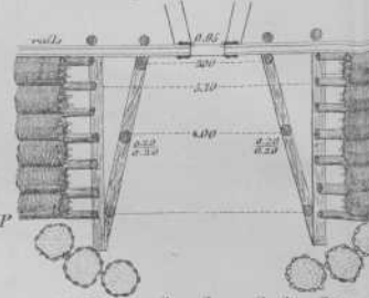
Fig. 18. Doorsnede volgens de lijn PQ van Fig. 17. (1:143)
