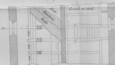
Fig. 20. Doorsnede volgens de lijn xy van Fig. 19. (1:143)
