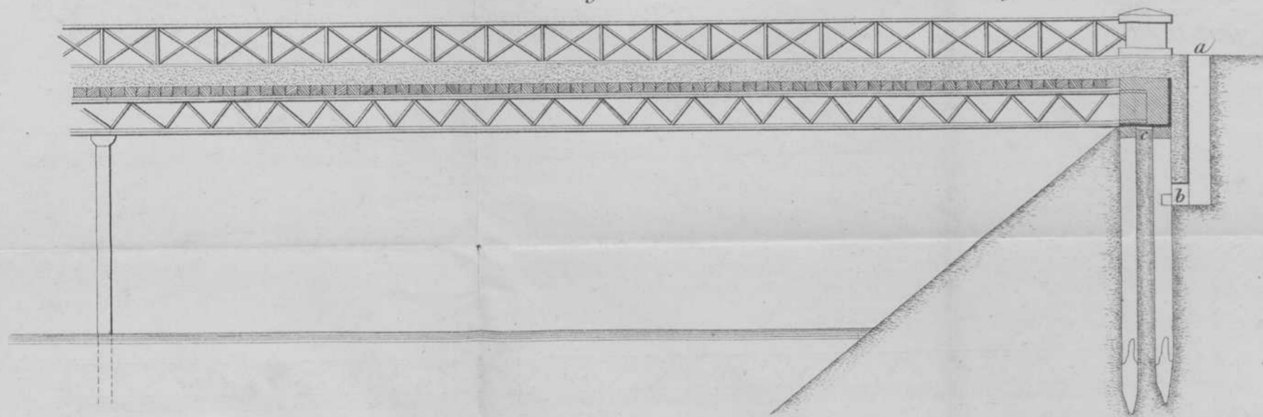
Fig. 4 b (1:200).
