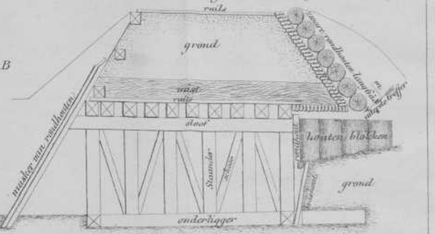
Fig. 14. Blindeering van Katharina. Plaatting der boorddekking van rails (1:100)
