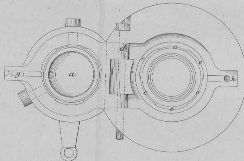
Achterlaadkanon van 7 tt . Het sluitstuk opgedraaid.
