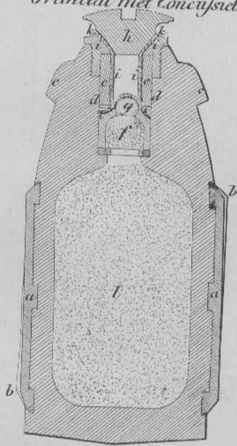
Fig. 3. Granaat met Concussiebuis.
