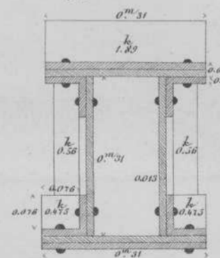
Fig. 6 (1:100).
