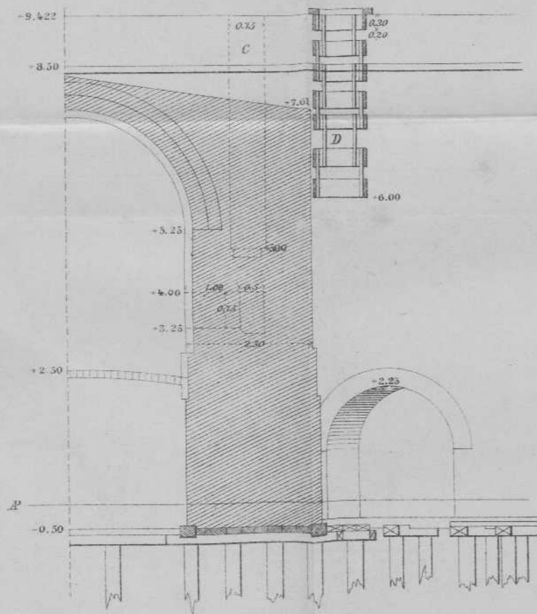
Fig. 2a (1:100)
