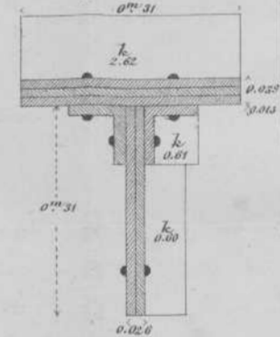
Fig. 7 (1:100).
