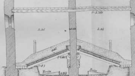
Fig. 20. Doorsnede volgens de lijn xy van Fig. 19. (1:143)
