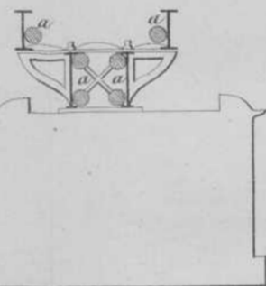
Systeem Schijfkorre en Howe. Fig. 5.
