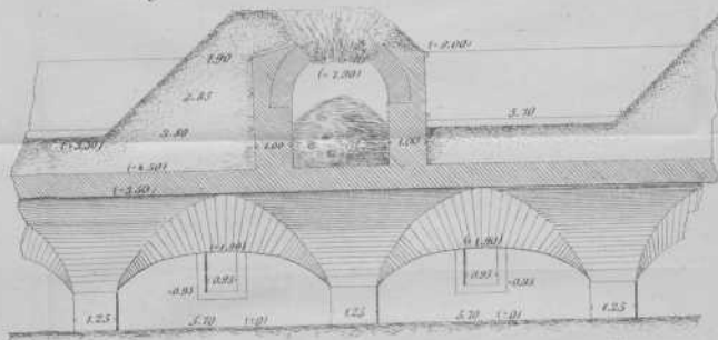
Fig. 12. Blindeering van Katharina. Doorsnede volgens de lijn CD van Fig. 14 en 16. (1:100)
