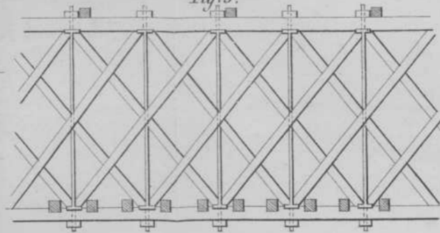
Systeem Schijfkorre en Howe. Fig. 5.
