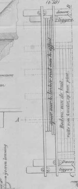
Fig. 21. Platte grond van een halve bedijing van rails met inzenking of knil voor de staart van het affuit. (1:50)
