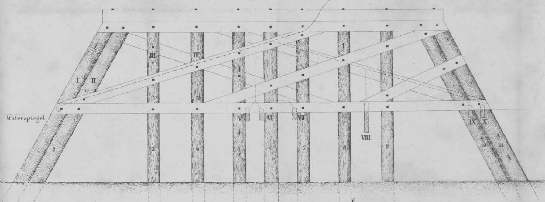
Fig. 2. (1:50)
