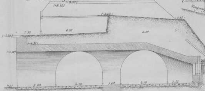
Fig. 10. Dwarsdoorsnede van Fig. 9. (1:143)
