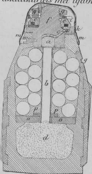
Fig. 4. Granaatkartets met tijdbuis.
