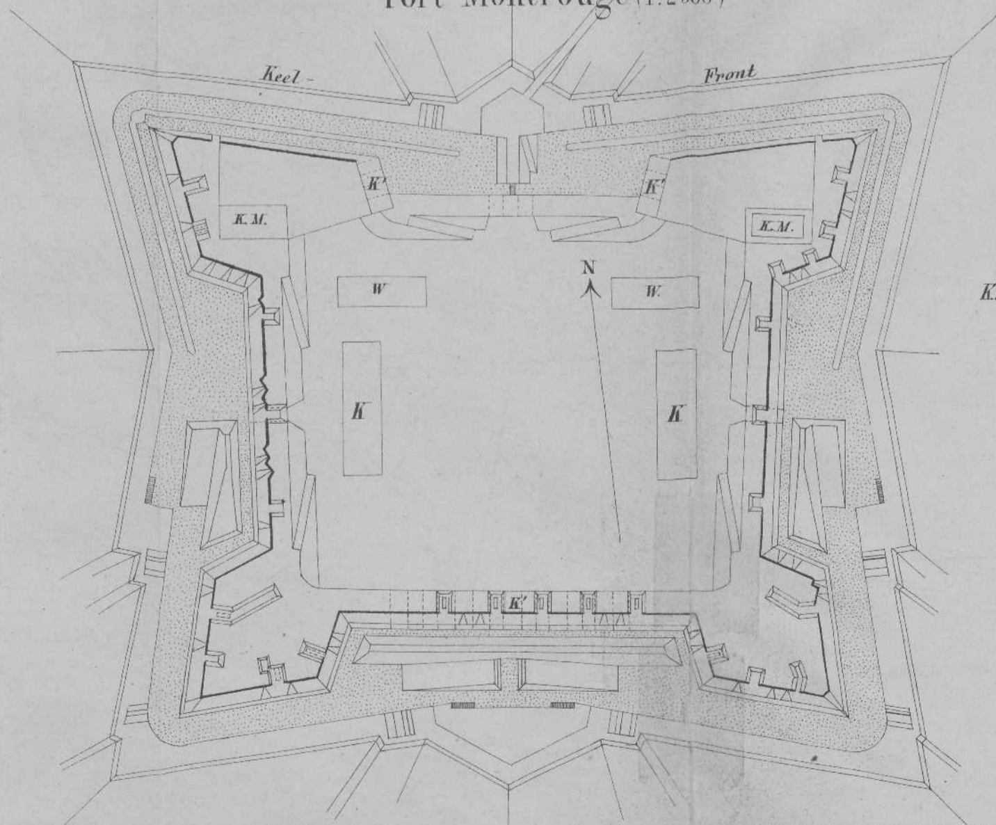
Fort Montrouge (1:2500)
