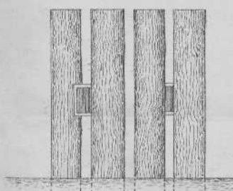
Fig. 3 a . (1:50)
