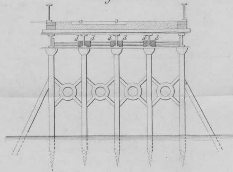
Fig. 3 a (1:100).
