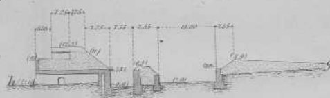
Fig. 6. Doorsnede volgens de lijn Am over de lage en hooge flank van het Bastion des Bourgeois (1:1200)
