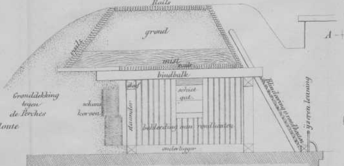
Fig. 22. Doorsnede volgens de lijn AB van Fig. 22. (1:50)
