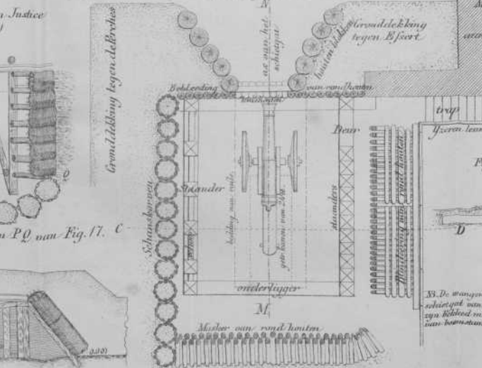
Fig. 16. Blindeering van Katharina. Platte grond (1:100)
