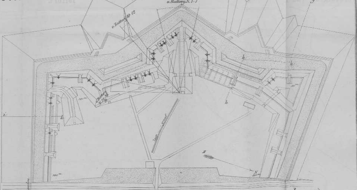
Fig. 2. Platte grond van het beheerscht door den, in't verlengde voorwaarts gelegen (ongeveer 1:2000)
