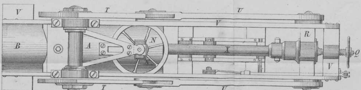
Fig. 4. Dwarshoofd met aangesloten palstaaf, van ter zijde gezien.
