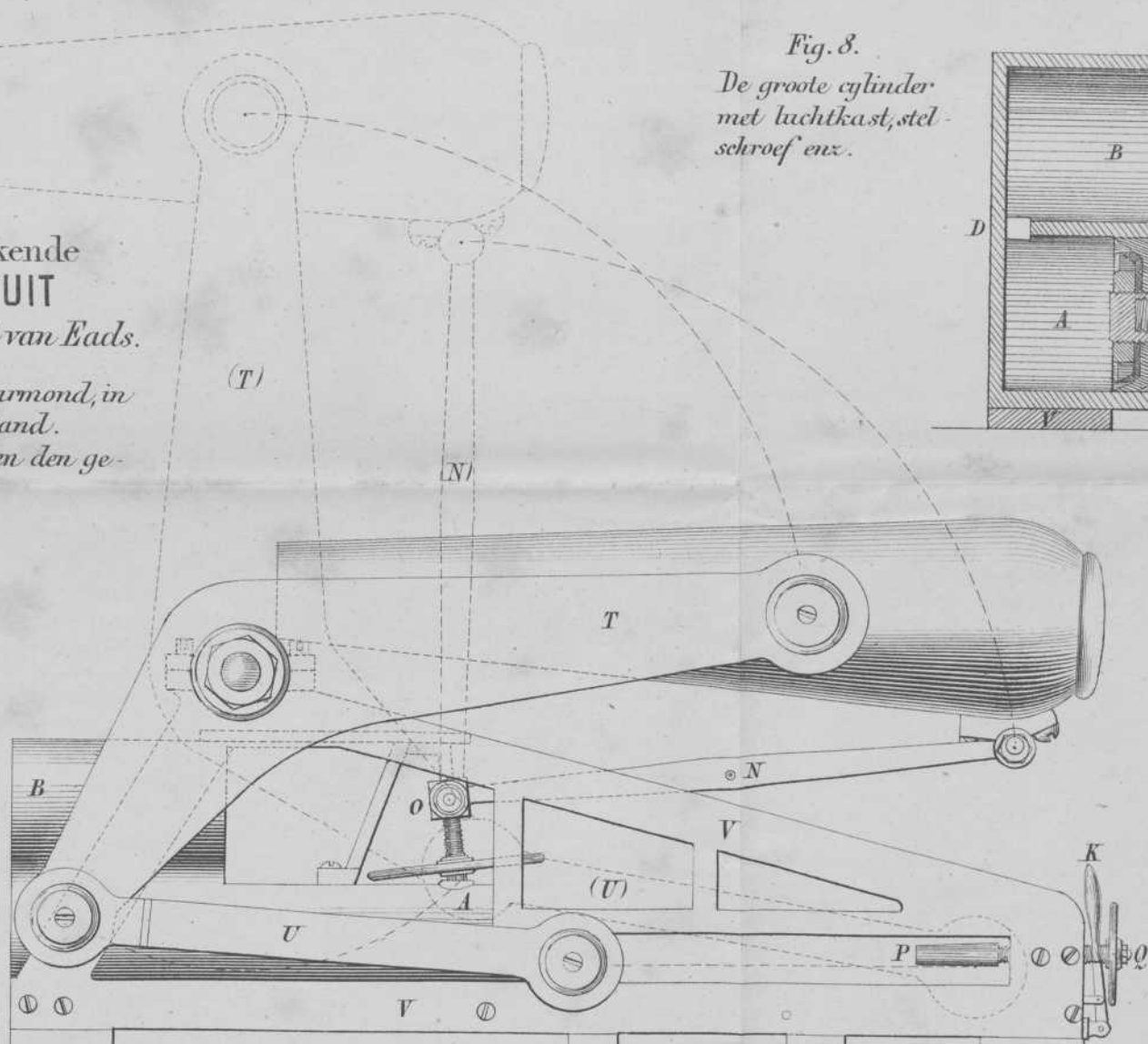
Fig. 3. De affuit, zonder den vuurmond, voor geheven stand voorgesteld.
