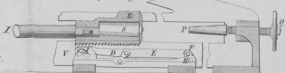
Fig. 7. Toestellen tot aandrukken en terug- trekken van den kniehefboom.
