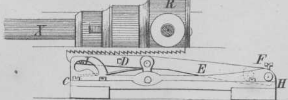
Fig. 6. Platte grond van de palstaaf, enz. (kniehefboom).
