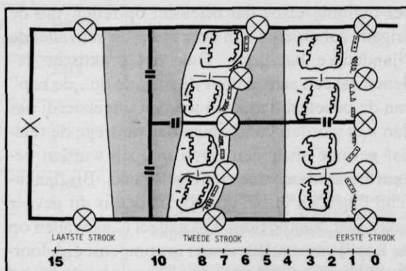
Afb. 8 De manoeuvreerterrein tussen de stroken; gerasterd: vrije manoeuvreerterrein nabij de stroken
