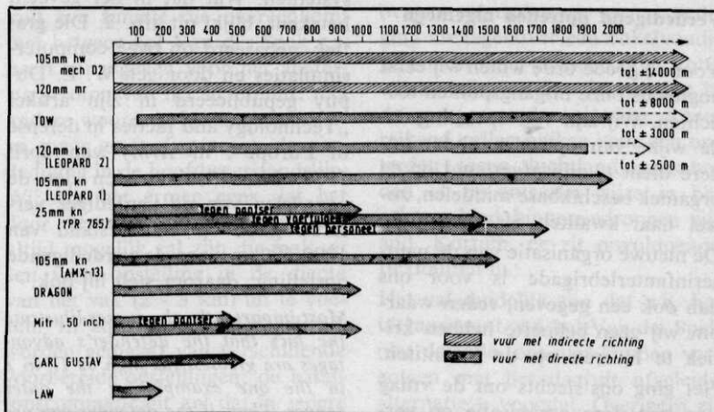
Afb. 1 Effectieve dracht van de belangrijkste wapensystemen, in te zetten uit een opstelling
