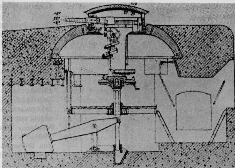
Afb. 23 Het inwendige van een hefkoepel
