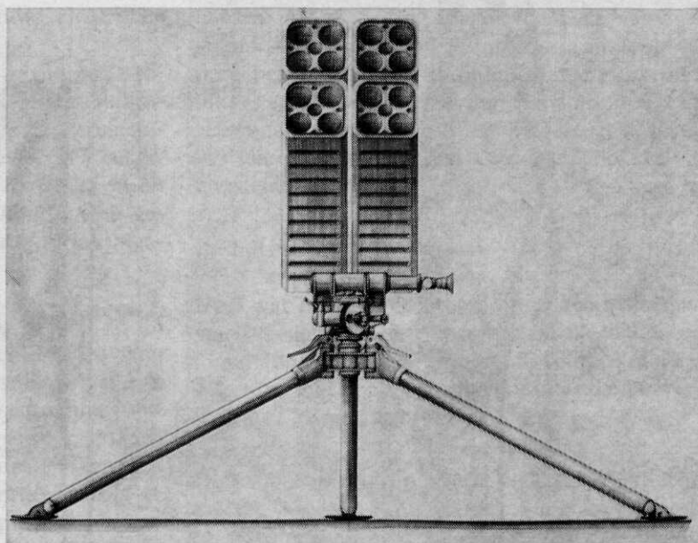
Rattlebox, tot vuren gereed; front-beeld
