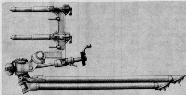
Rattlebox-affuit, samengeklapt, zonder lanceerbuizen
