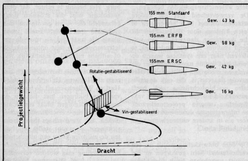
Afb. 1 Relatie projectielgewicht—dracht
