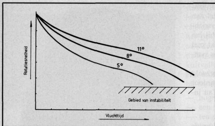
Afb. 6 Rotatieafneming bij verschillende nokkenstanden
