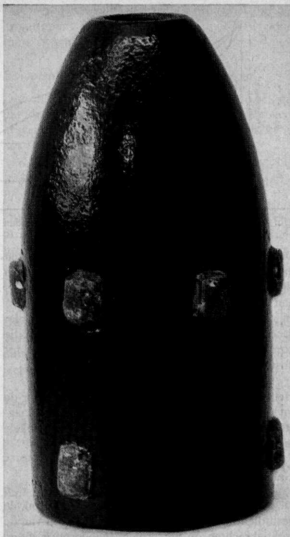
Afb. 5 Nokkenprojectiel 16 cm, voorlader
