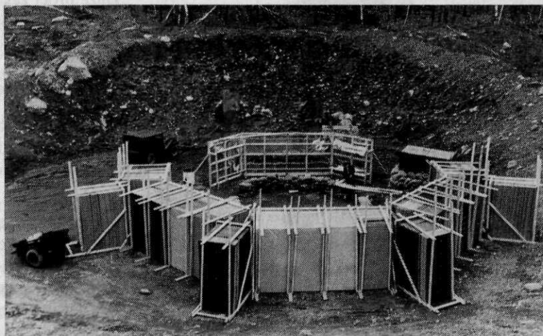
Afb. 8 Arena voor springproeven
