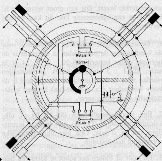
Afb. 17 Stabilisatie-inrichting
