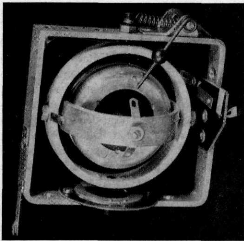
Afb. 16 Gyroscoop met sleepcontact
