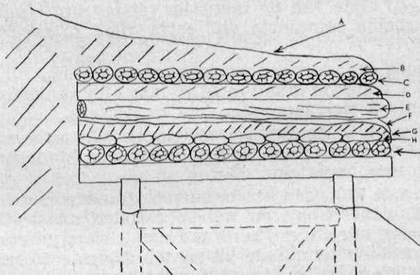
Afb. 2 Bovendekking van een bunker
