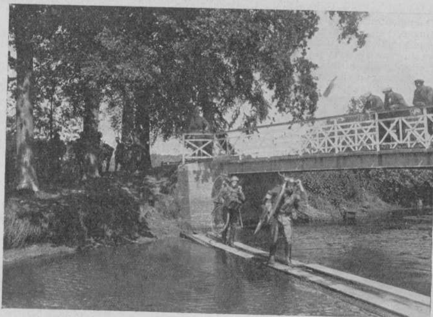
Afb. 3. Het gebruik van de kratbrug.
