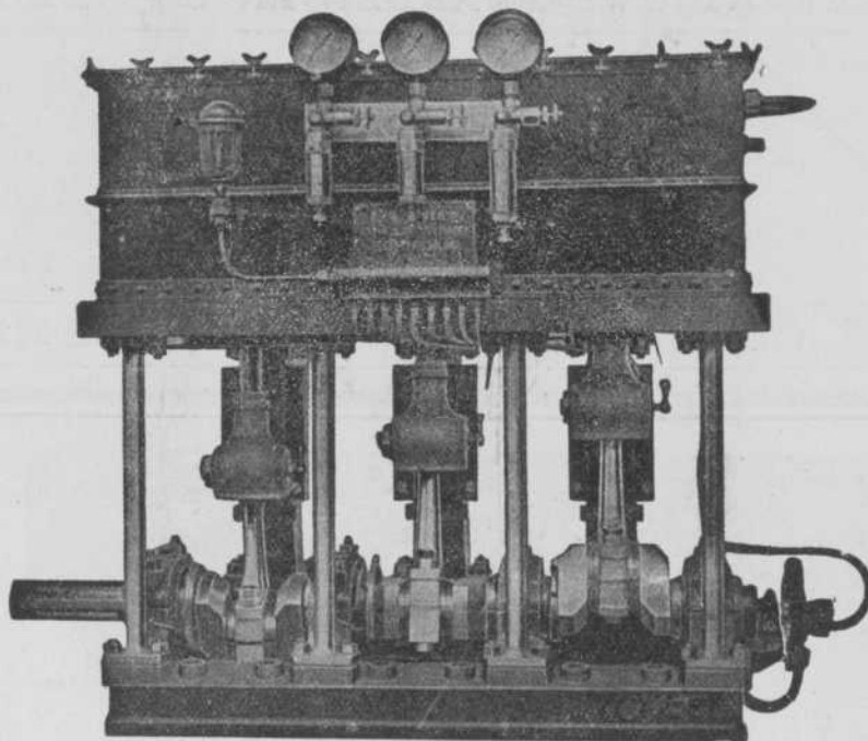
Drietredige snelloopende Luchtcompressor voor marine doeleinden 200 Atm.
