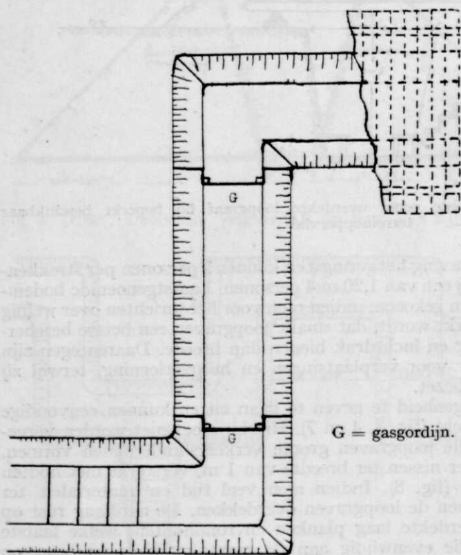
Fig. 9 (1:75). Overdekte loopgraaf met gasluis en gebroken ingang.
