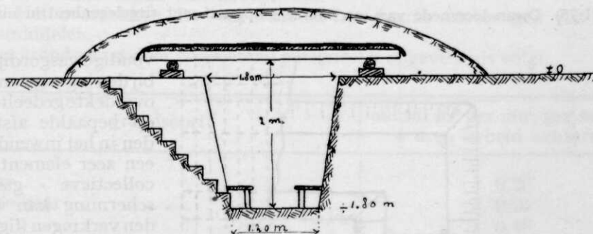
Fig. 7 (1:75). Dwarsdoorsnede eener overdekte loopgraaf bij beperkt beschikbaar terreinoppervlak.
