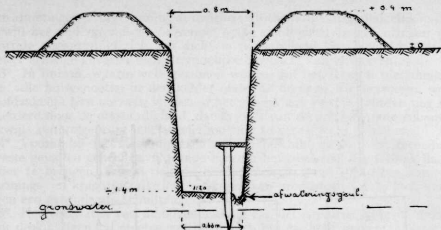
Fig. 3. (1:37 1/2). Doorsnede volgens AB op fign. 1 en 2 (bij lagen grondwaterstand).
