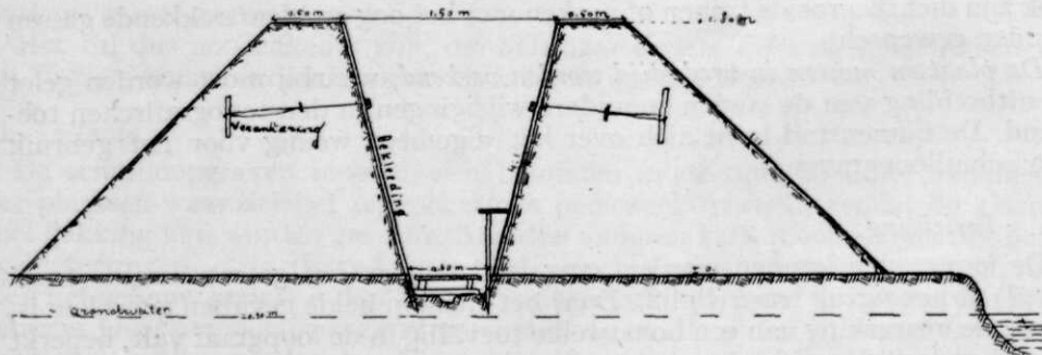
Fig. 4. (1:60). Doorsnede volgens AB op fign. 1 en 2 (bij hoogen grondwaterstand.)
