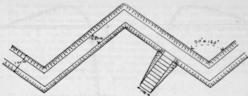
Fig. 6. (1:150). Plattegrond van een loopgraaf bij onbeperkt beschikbaar terrein-oppervlak (zig-zag tracé).
