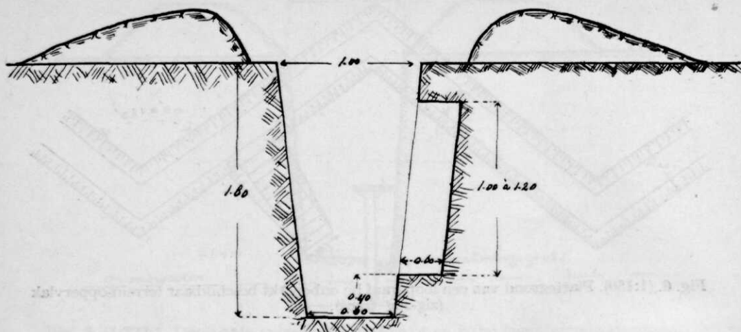
Fig. 8. (1:75). Dwarsdoorsnede van een smalle loopgraaf met zitgelegenheid in nissen.
