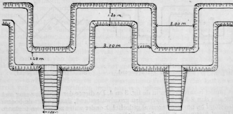
Fig. 5 (1:150). Plattegrond van een loopgraaf bij beperkt beschikbaar terreinoppervlak (getraverseerd tracé).
