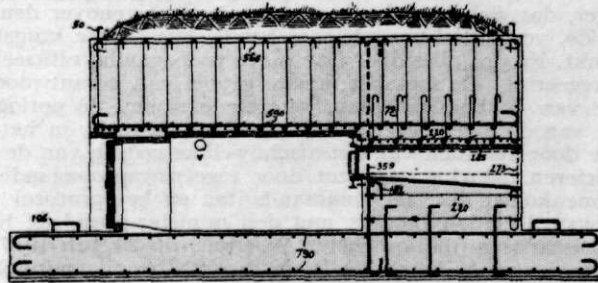
Afb. 3. Doorsnede volgens CD op afb. 1. Schaal 1:100.
