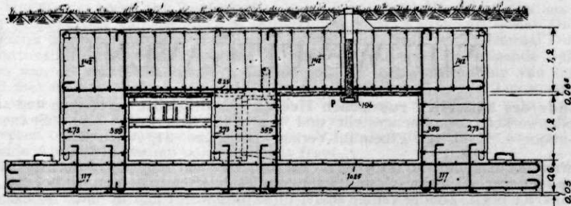
Afb. 2. Doorsnede volgens AB op afb. 1. Schaal 1:100.
