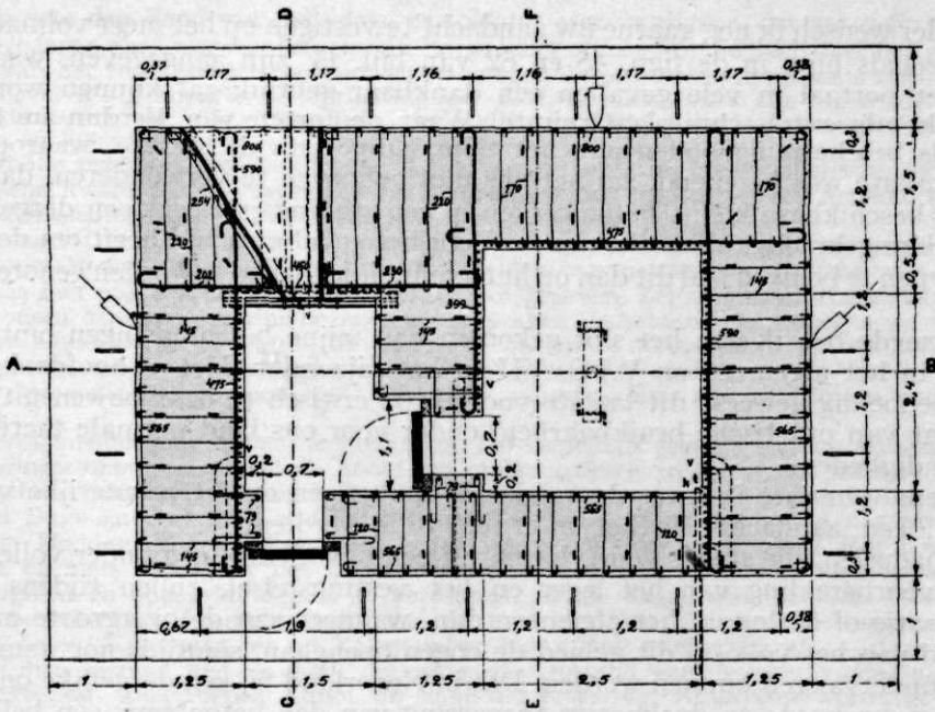
Afb. 1. Plattegrond. Schaal 1:100.
