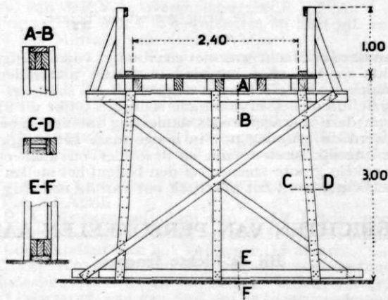
Afb. 1. Constructie van de schragen.
