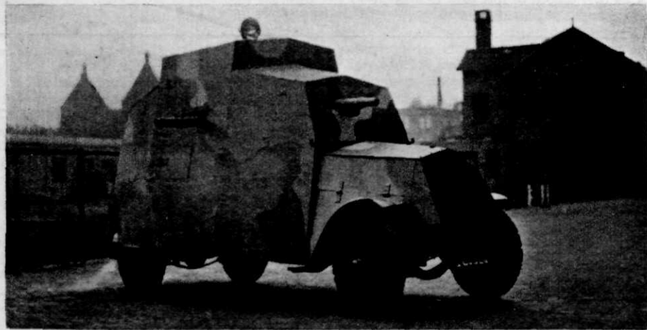
Afb. 1. Een der pantserwagens, gebouwd in de werkplaatsen van de Schoolcompagnie van den Motordienst te Haarlem, op G. M. C.-automobielen
