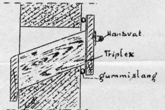
Gasstop voor schiet gat.
