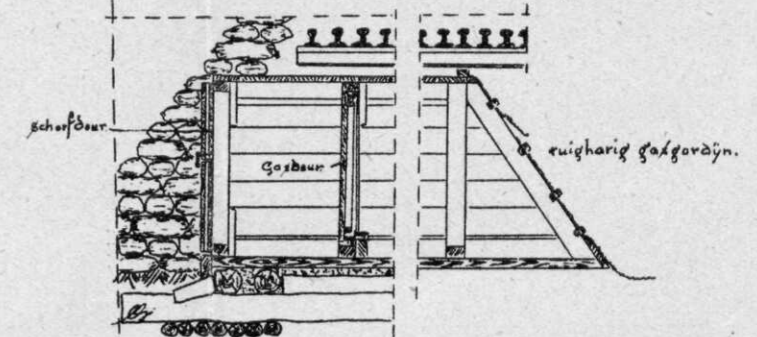
Gasfluis voor granatruye schuilplaats.
