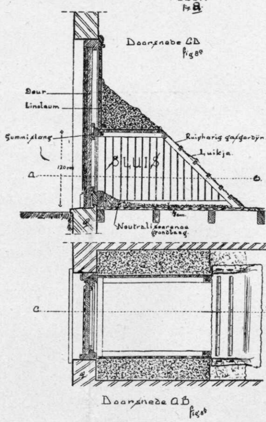
Gasdichte afsluiting van een naar buiten draaiende deur.
