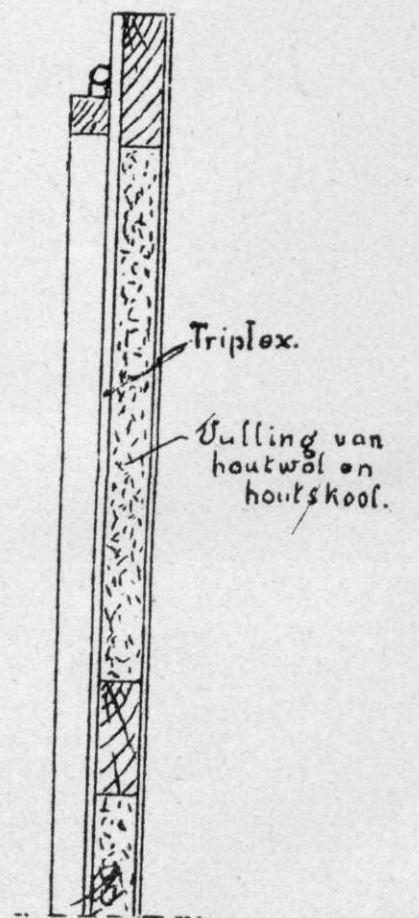
Gasstop voor schiet gat.
