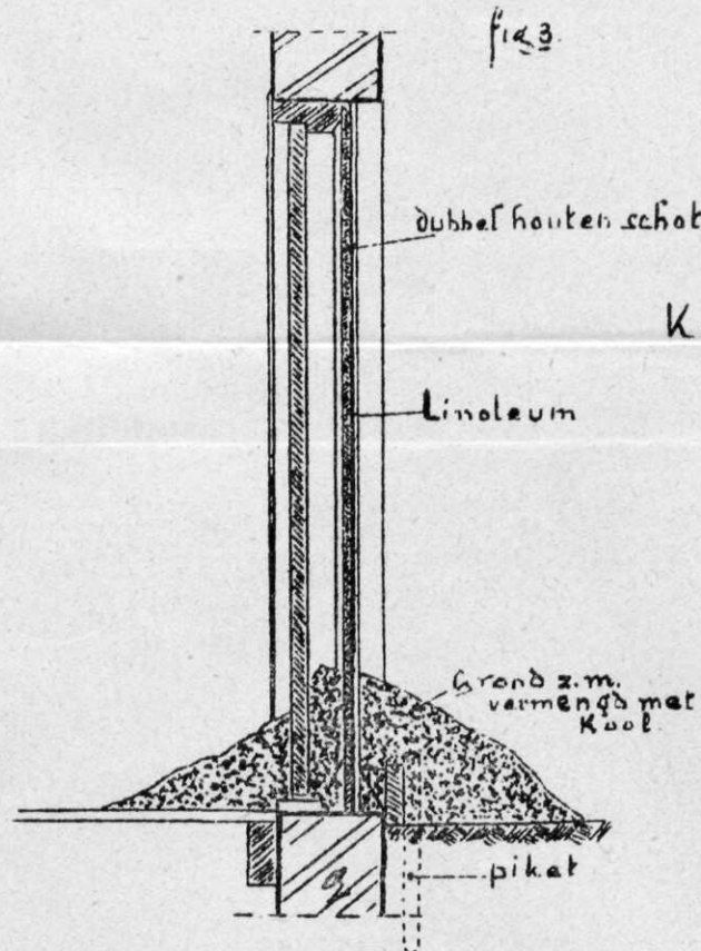
Gasdichte afsluiting van een naar binnen draaiende gangbare deur.
