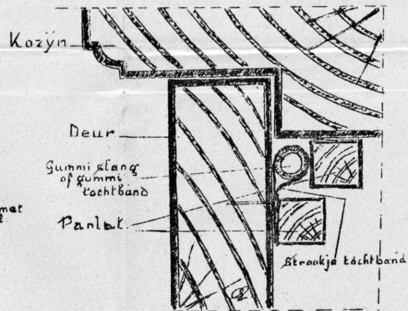
Gasdichte afsluiting van een naar binnen draaiende gangbare deur.
