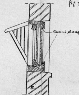
Gasdichte afsluiting van een gangbare dubbele deur.
