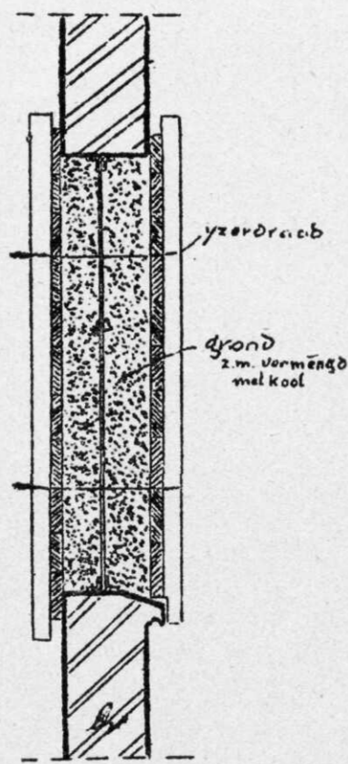
Gasdichte afsluiting van een raam met yzeren kozyn.
