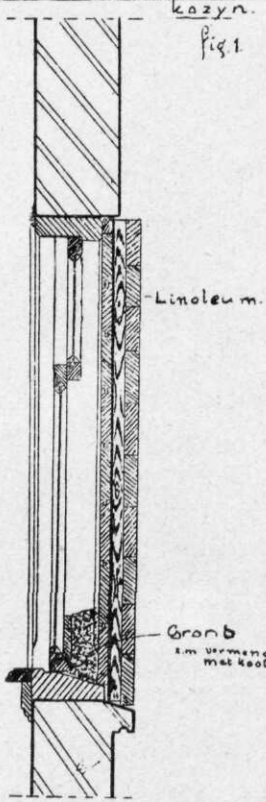
Gasdichte afsluiting van een raam met houten kozyn.
