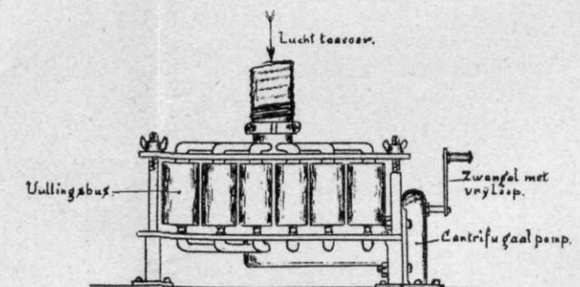
Luchtfilter voor 12 personen.
