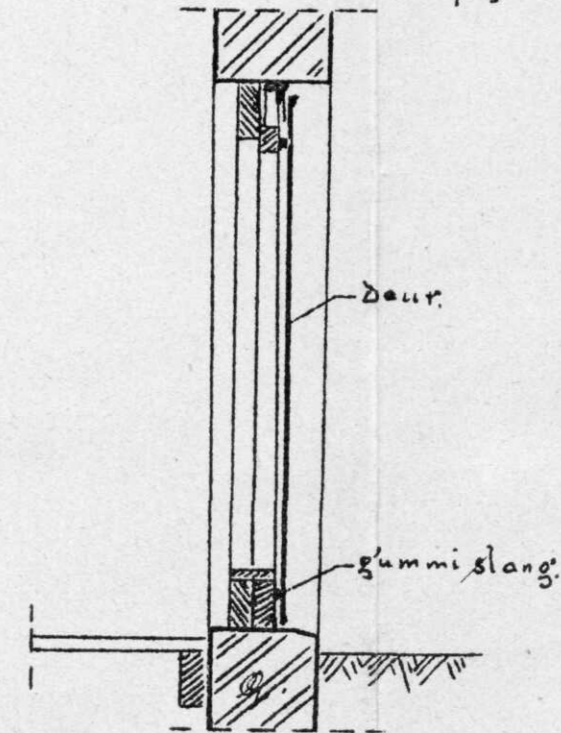
Gasdichte afsluiting van een gangbare stalen deur.
