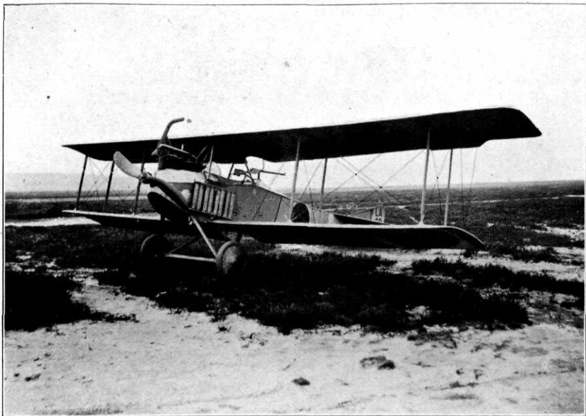
Verkenningvliegtuig type L(uft)-, V(erkehr)-, G(esellschaft), bewapend met 1 mitrailleur.
