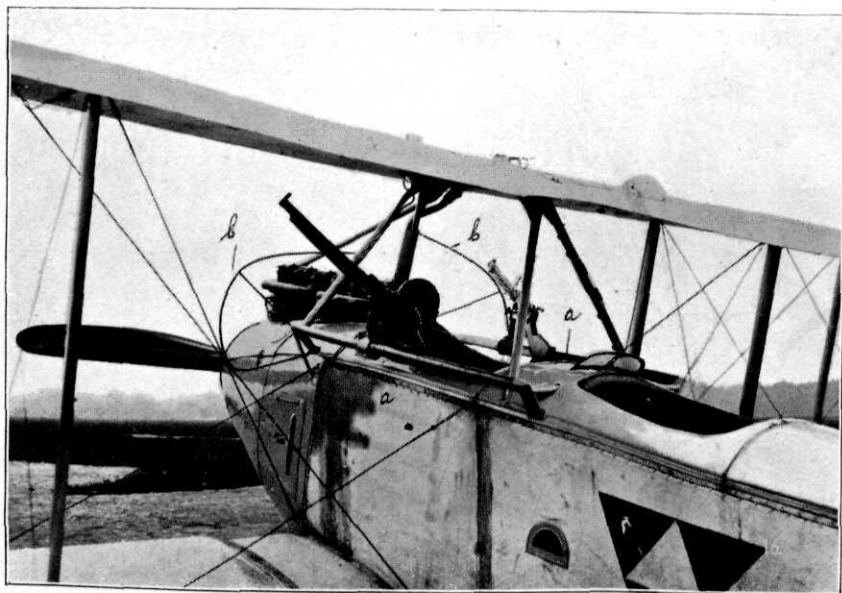
Voorste gedeelte van een verkenningsvliegtuig, type Aviatik.
