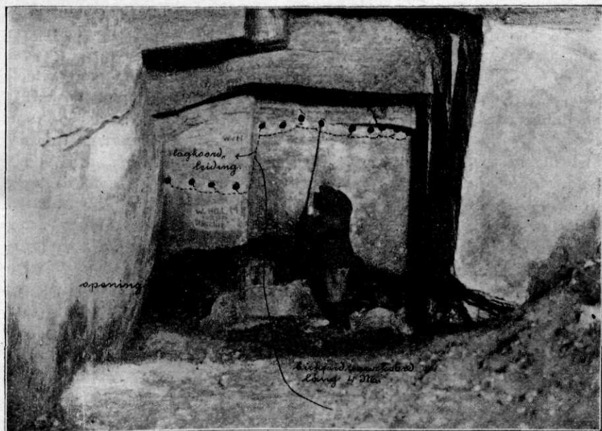
Fig. 7. Plaats van de ladingen bij den tweeden toegang.
