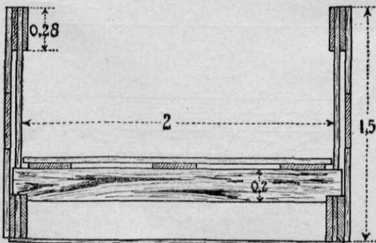
Figuur 2. Dwarsdoorsnede volgens A—B.
