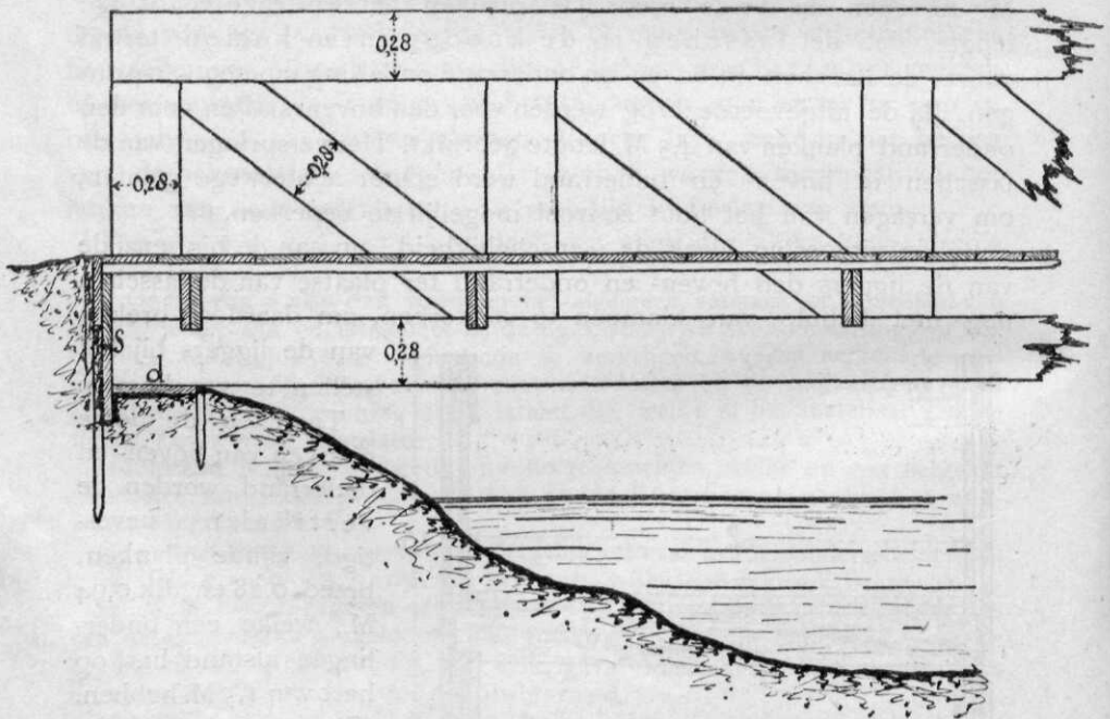
Figuur 4. Lengtedoorsnede.
