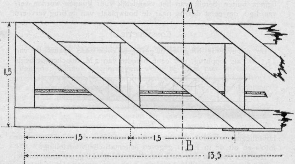
Figuur 3. Zijaanzicht.
