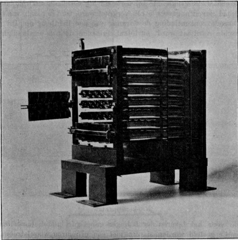
Leidsche flesschenbatterij.
