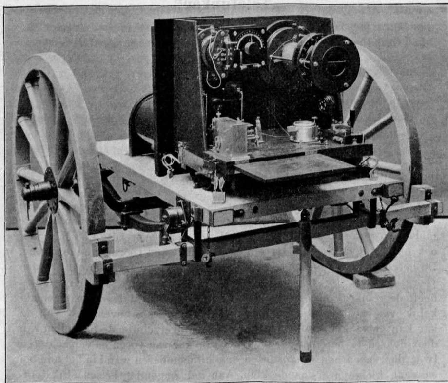
TOESTELKAR.
