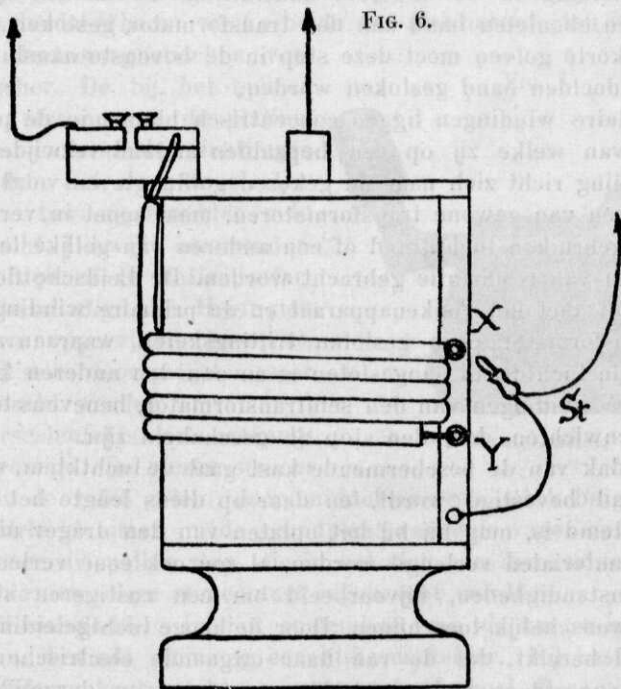
Hooge-spannings-transformator.
