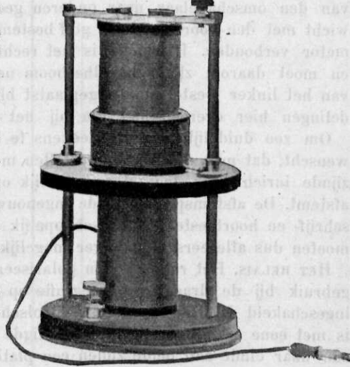
Ontvangstransformator.
