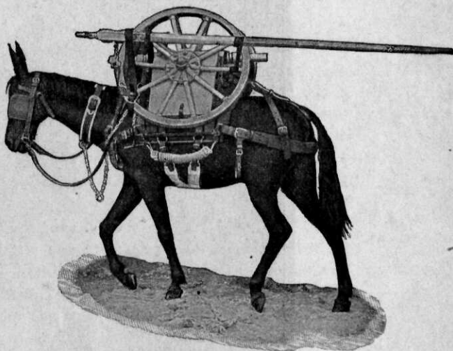
FIG. 9. Affuitas met raden, disselboom, twee kisten tot onderdeelen en eenig toebehooren.
