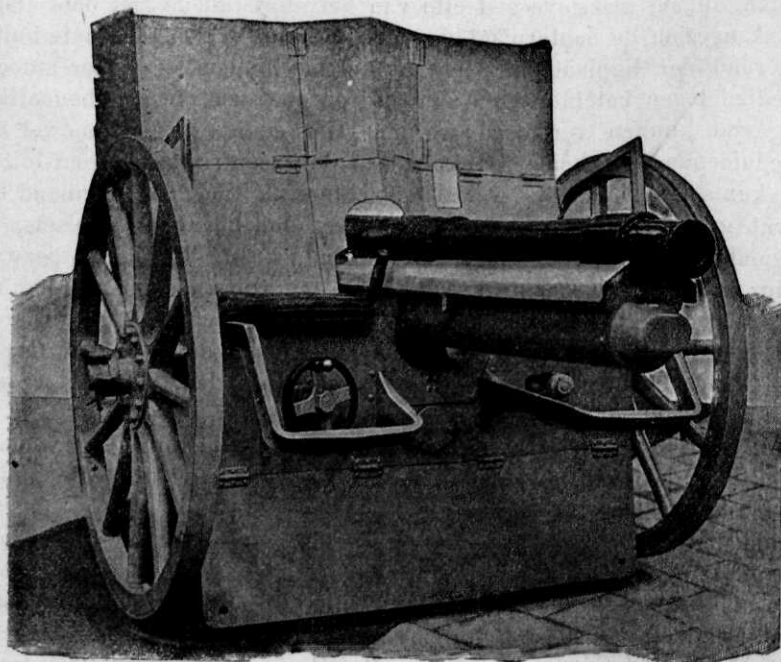
FIG. 4. Snelvuurveldgeschut, stelsel EHRHARDT, met „Kammverschluss" en opklapbaar pantserschild.
